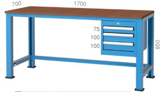
3110 700 X 1700 X 850 mm
