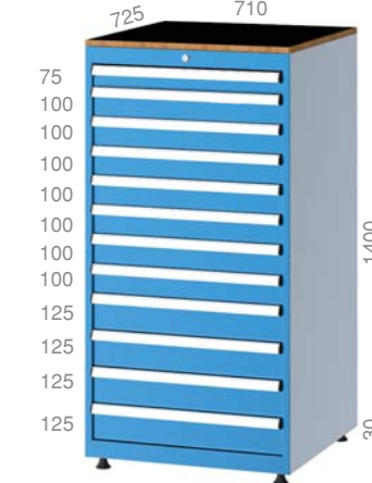
7401 725 X 710 X 1430 mm
