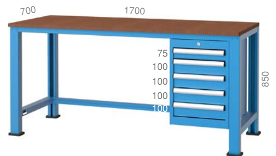
3120 700 X 1700 X 850 mm
