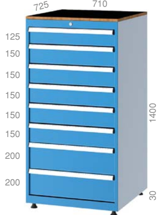
7402 725 X 710 X 1430 mm
