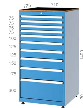
7400 725 X 710 X 1430 mm
