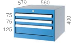
5041 570 X 560 X 400 mm
