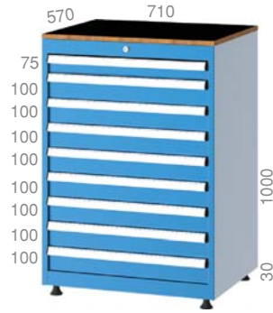
75101 570 X 710 X 1030 mm
