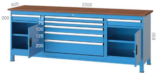
3642 600 X 2200 X 850 mm
