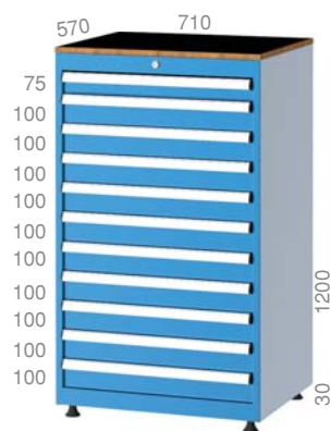
75201 570 X 710 X 1230 mm
