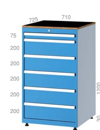
7202 725 X 710 X 1230 mm
