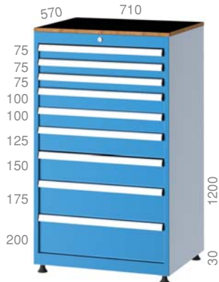
75200 570 X 710 X 1230 mm
