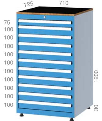
7201 725 X 710 X 1230 mm
