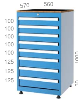
5101 570 X 560 X 1030 mm
