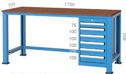
3131 700 X 1700 X 850 mm
